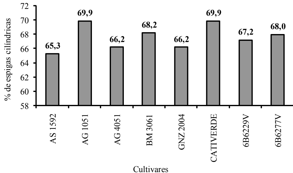
FIGURA 2. Porcentagem de espigas cilíndricas em oito cultivares de milho verde, avaliadas em Campinas, Mococa e Capão Bonito, na safrinha de 2009.
